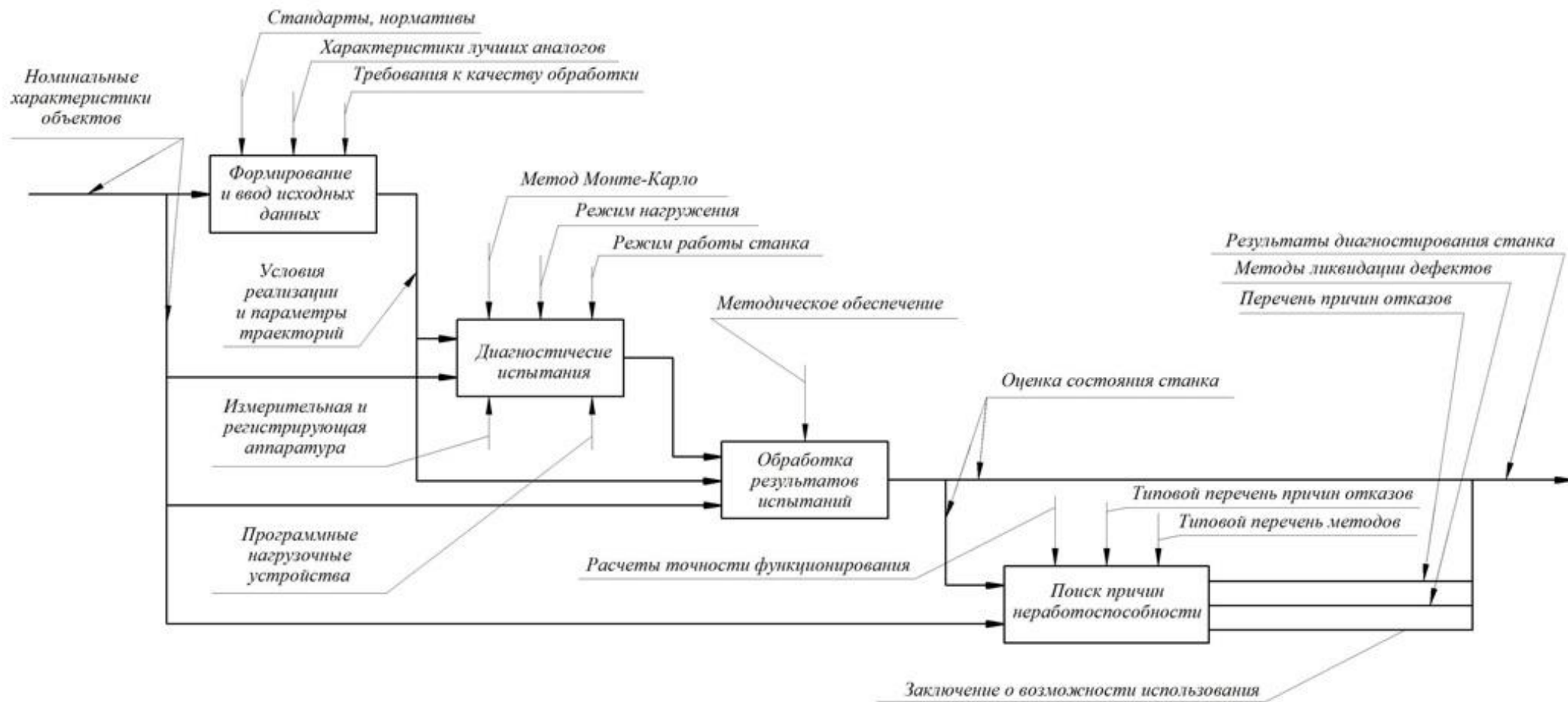
Рис 2. Структурная диаграмма типовой методики диагностирования.
