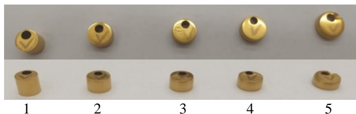
Рис.1. Образцы с износостойким покрытием TiN 1 - \varepsilon = 0\% ; 2 - \varepsilon = 20\% ; 3 - \varepsilon = 26\% ; 4 - \varepsilon = 36\% ; 5 - \varepsilon = 46\%
