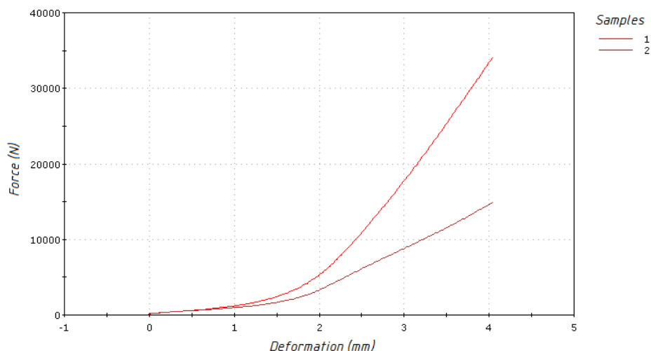
Рис. 2. Зависимости изменение силы осадки от перемещения (1 – композитный образец, 2 – полиуретановый образец)
