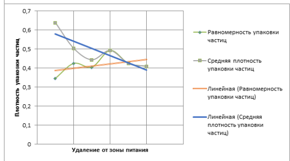
Упаковка в повороте на 90 град.
