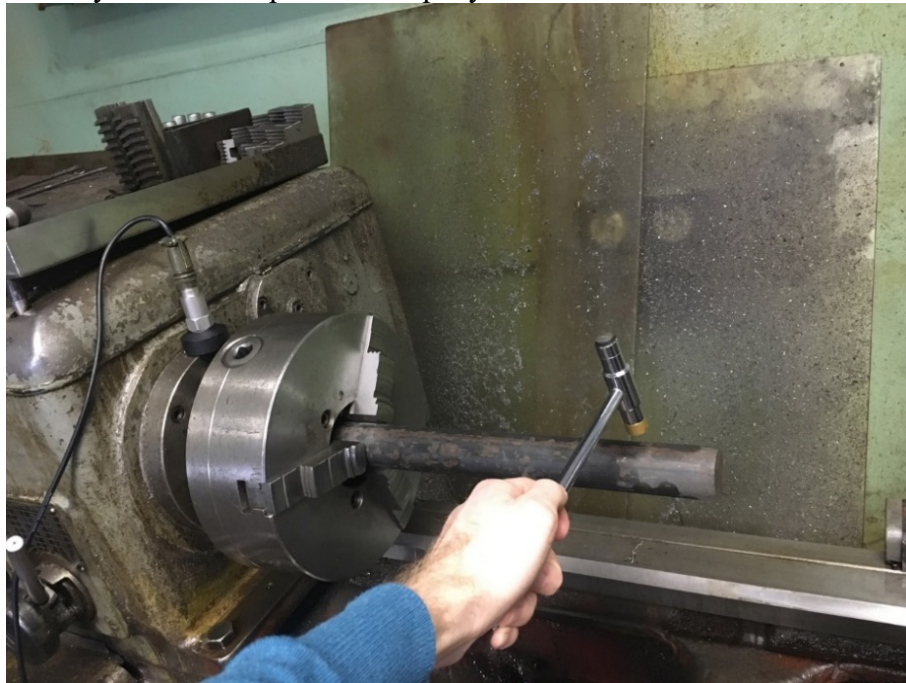
Рисунок 4 – Проведение статических испытаний
