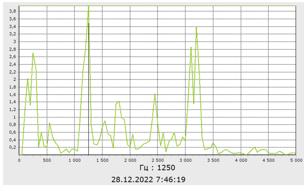
Рисунок 6 - Спектр колебаний системы с прутком, имеющим дефект
