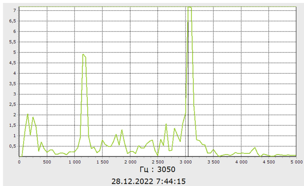
Рисунок 5 – Спектр колебаний системы с целым прутком
