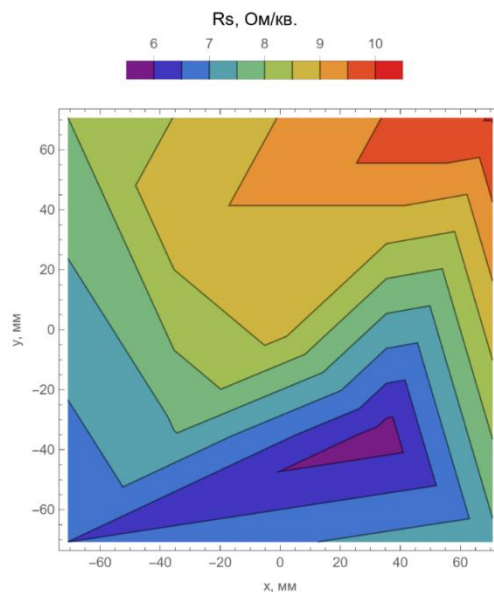
Рис. 2 Зависимость поверхностного сопротивления от удаления от центра подложкодержателя
