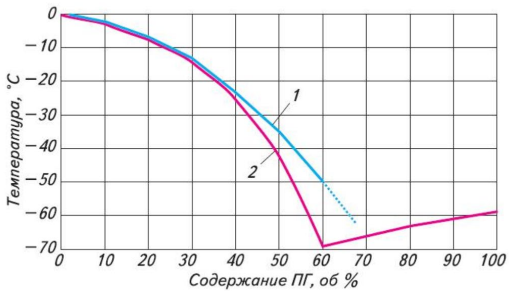
Рис. 1. Зависимость температур начала кристаллообразования t_{\text{н.кр}} (1) и замерзания t_{\text{зам}} (2) от концентрации пропиленгликоля (ПГ) в воде
