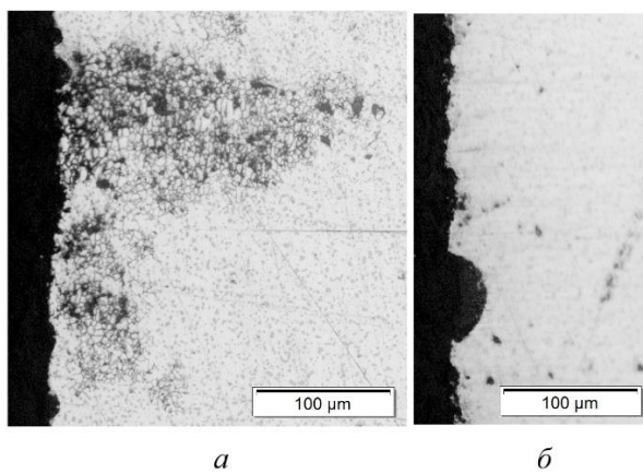
Рис.2. Коррозионные поражения после ускоренного испытания на МКК (x200) а – закалка, б – закалка и искусственное старение (30 часов)
