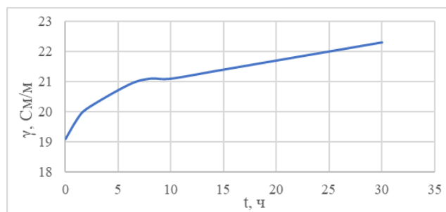
Рис. 1. Зависимость удельной проводимости от времени старения
