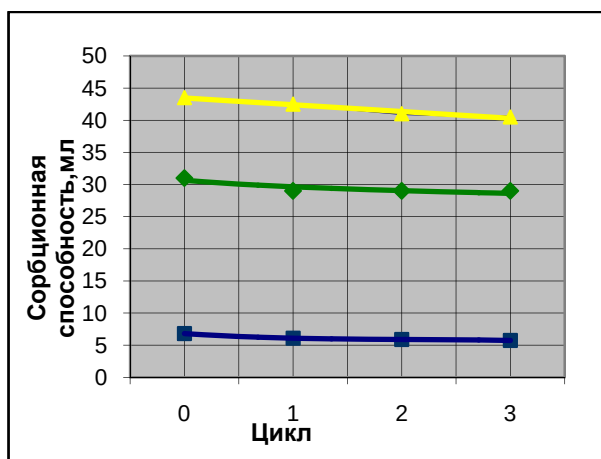
Рис. 2.2. Зависимость сорбционной способности ПГС от числа термических циклов
