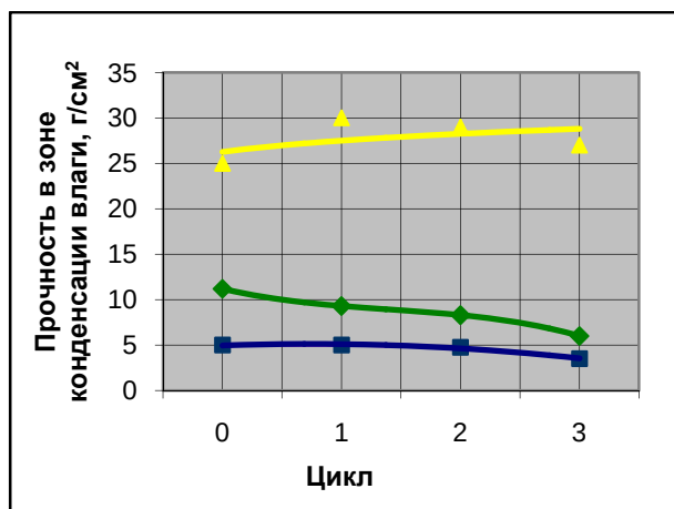
Рис. 1.1. Зависимость прочности при сжатии во влажном состоянии от числа термических циклов
