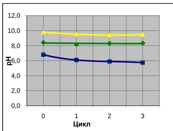
Рис. 2.1. Зависимость водородного показателя ПГС от числа термических циклов
