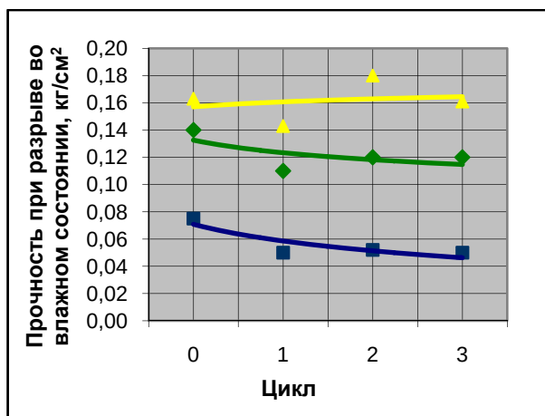
Рис. 1.2. Зависимость прочности при разрыве во влажном состоянии от числа термических циклов
