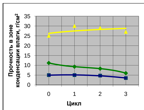
Рис. 1.4. Зависимость прочности в зоне конденсации влаги от числа термических циклов
