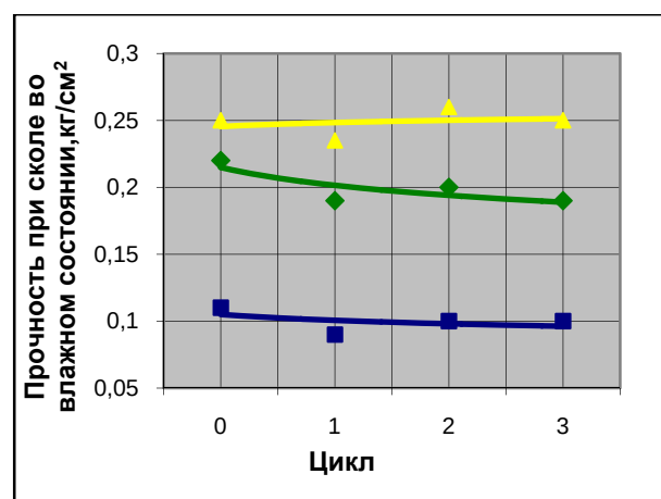
Рис. 1.3. Зависимость прочности при сколе во влажном состоянии от числа термических циклов
